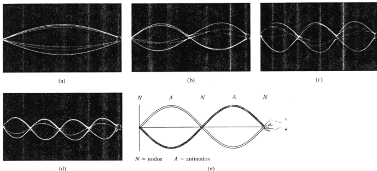
15.20 (a)–(d) Exposiciones sucesivas de ondas estacionarias en una cuerda estirada. De (a) a (d), la frecuencia de oscilación del extremo derecho aumenta, y la longitud de la onda estacionaria disminuye. (e) Los extremos del movimiento de la onda estacionaria de (b), con nodos en el centro y en los extremos. El extremo derecho de la cuerda se mueve muy poco en comparación con los antinodos, así que es prácticamente un nodo.
