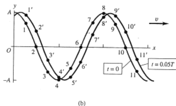
15.7 (a) Otra vista de la onda en t = 0 de la figura 15.6a. Los vectores muestran la velocidad transversal v_y y la aceleración transversal a_y en varios puntos de la cuerda. (b) Las dos curvas muestran la onda en t = 0 y en t = 0.05T . Durante este intervalo, una partícula en el punto 1 se desplaza al punto 1', una partícula en el punto 2 se desplaza al punto 2', etcétera.
