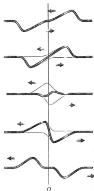
15.17 Traslape de dos pulsos de onda —uno hacia arriba, el otro invertido— que viajan en direcciones opuestas. El tiempo aumenta hacia abajo.
