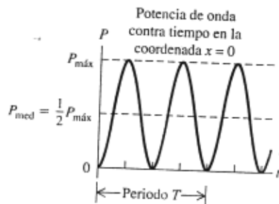
15.13 La potencia instantánea P(x, t) de una onda senoidal, dada por la ecuación (15.23), se muestra en función del tiempo en la coordenada x = 0 . La potencia nunca es negativa, lo que implica que la energía nunca fluye en dirección opuesta a la de propagación de la onda.
