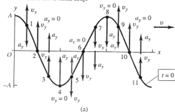
15.7 (a) Otra vista de la onda en t = 0 de la figura 15.6a. Los vectores muestran la velocidad transversal v_y y la aceleración transversal a_y en varios puntos de la cuerda. (b) Las dos curvas muestran la onda en t = 0 y en t = 0.05T . Durante este intervalo, una partícula en el punto 1 se desplaza al punto 1', una partícula en el punto 2 se desplaza al punto 2', etcétera.
