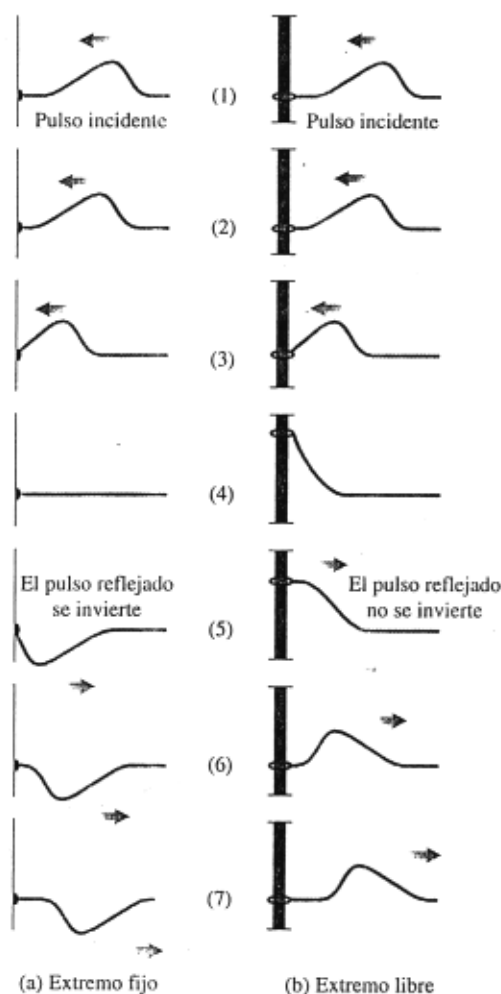
15.16 Reflexión de un pulso de onda (a) en un extremo fijo de una cuerda y (b) en un extremo libre. El tiempo aumenta hacia abajo.
