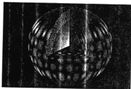
15.24 Los astrónomos han descubierto que el Sol oscila en varios modos normales distintos. En esta simulación en computadora de uno de esos modos, el azul denota lugares en los que el material solar se mueve hacia afuera; el rojo indica dónde se mueve hacia adentro.
