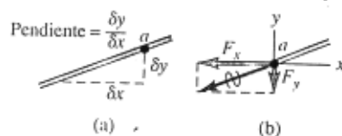
15.12 (a) Punto a en una cuerda que lleva una onda de izquierda a derecha. (b) Componentes de la fuerza ejercida sobre la parte derecha de la cuerda por la parte izquierda en el punto a .
