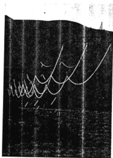
15.9 Estos cables tienen una cantidad relativamente grande de masa por unidad de longitud ( \mu ) y una tensión ( F ) baja. Si los cables sufren una perturbación (como cuando un ave se posa sobre ellos), viajarán ondas transversales en ellos con rapidez baja v = \sqrt{F/\mu} .
