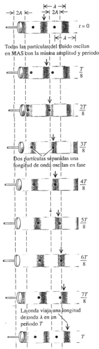
15.5 Onda senoidal longitudinal que viaja a la derecha por un fluido. La onda tiene la misma amplitud y periodo que la oscilación del pistón. Los puntos azul y rojo representan partículas del fluido cuyas coordenadas x difieren en la longitud de onda \lambda . En equilibrio, la partícula representada por el punto rojo está a \frac{1}{2} longitud de onda del pistón; sus oscilaciones están defasadas medio ciclo respecto al pistón.
