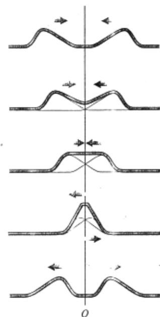
15.18 Traslape de dos pulsos de onda —ambos arriba de la cuerda— que viajan en direcciones opuestas. El tiempo aumenta hacia abajo.
