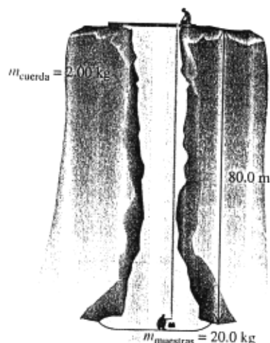
15.11 Envío de señales mediante ondas transversales en una cuerda vertical.
