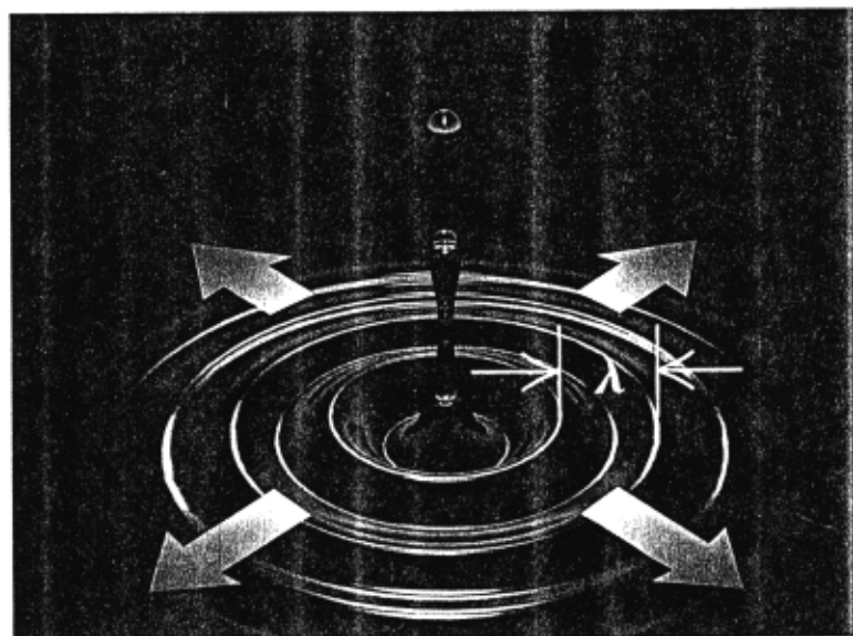
15.4 Una serie de gotas que cae en agua produce una onda periódica que se extiende radialmente hacia afuera. Las crestas y valles de la onda son círculos concéntricos. La longitud de onda \lambda es la distancia radial entre crestas adyacentes o valles adyacentes.
